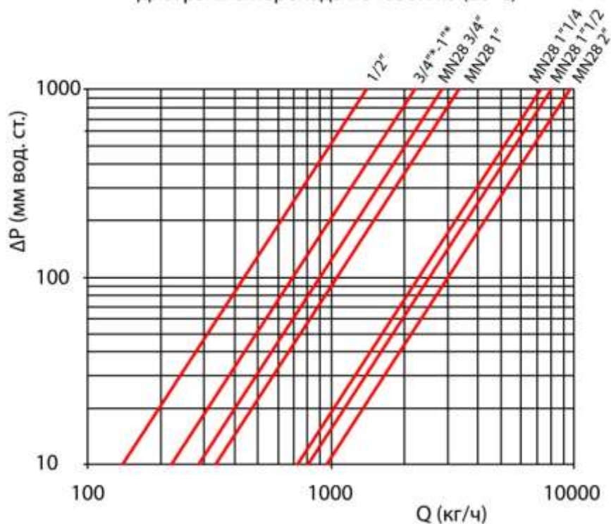
Диаграмма перепада по нефти (вязкость \leq 3^\circ E )
