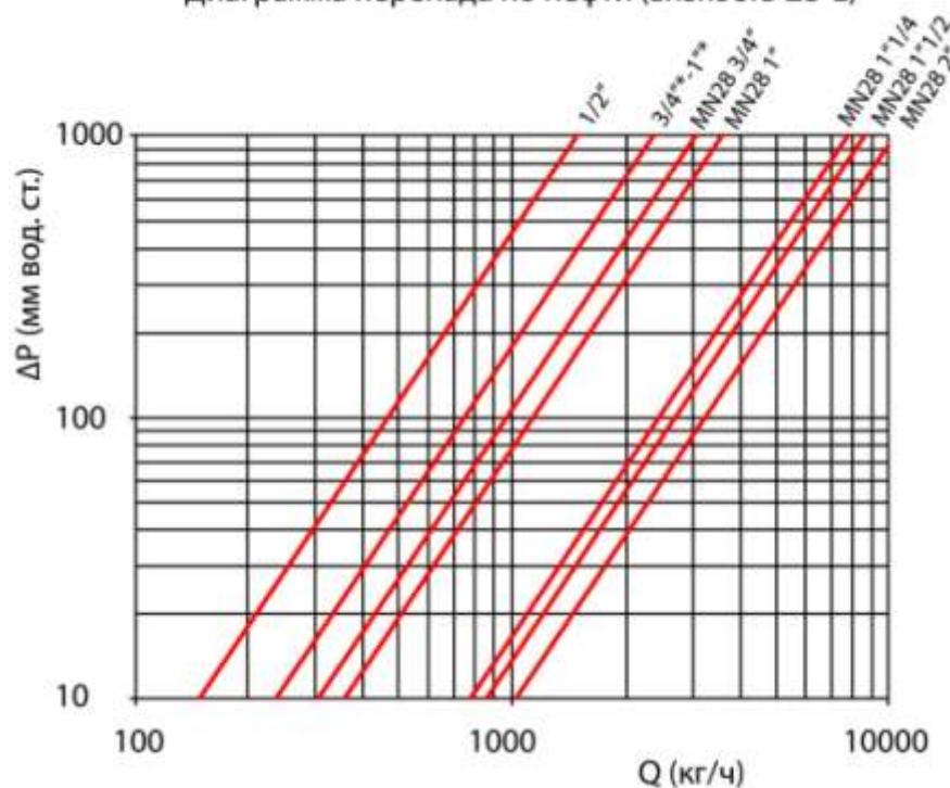
Диаграмма перепада по нефти (вязкость \leq 3^\circ E )
